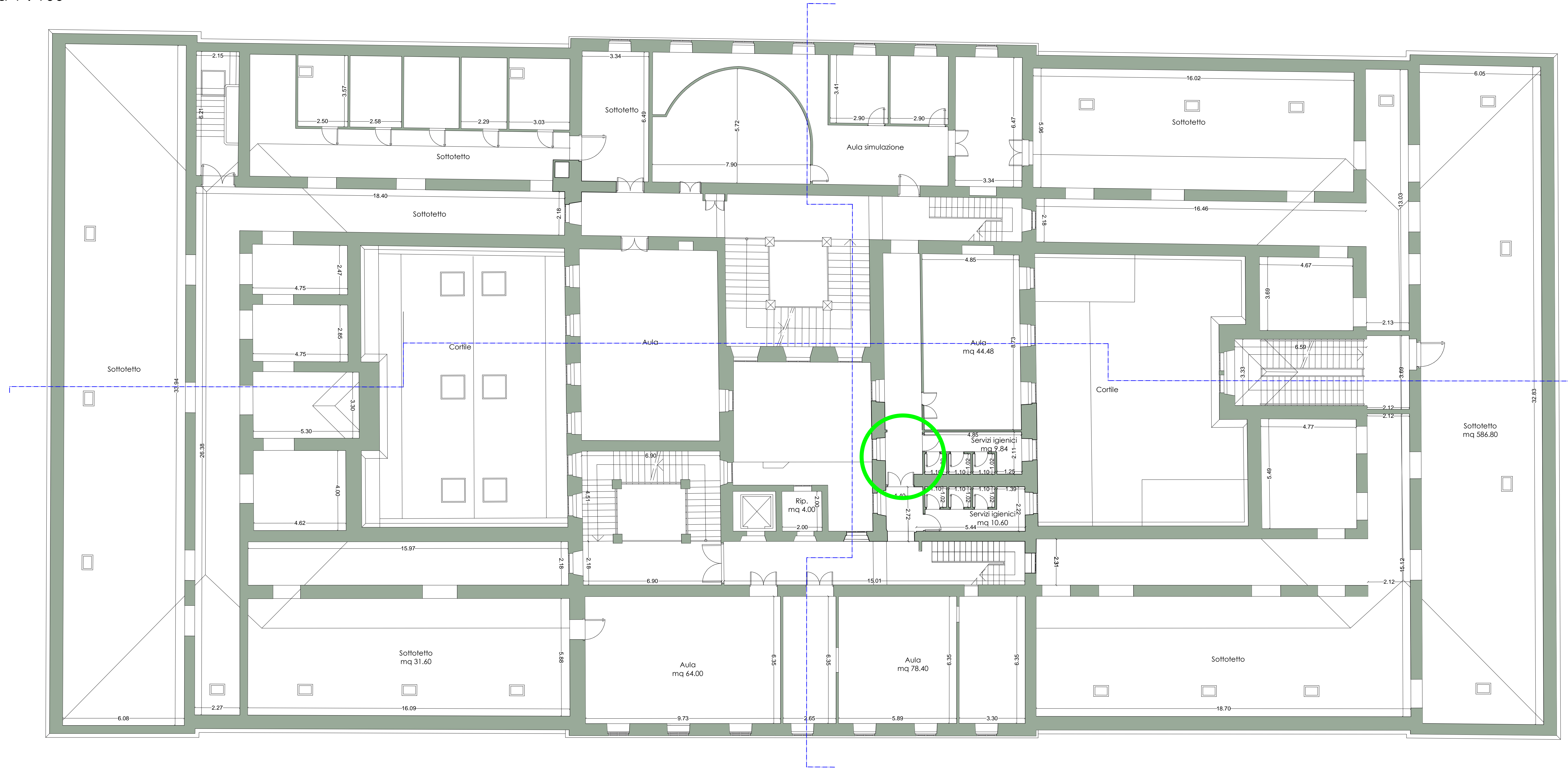
PLANIMETRIA QUARTO PIANO - stato di fatto Scala 1 : 100
