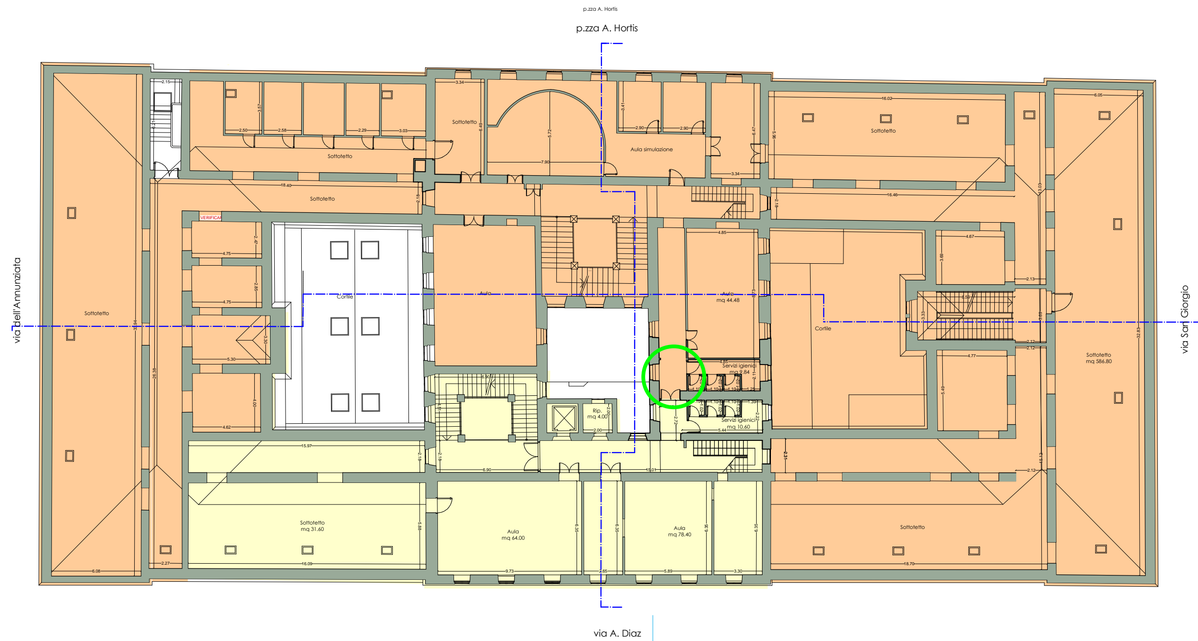
PLANIMETRIA QUARTO PIANO - stato di fatto Individuazione sedi ITC e ITN Scala 1 : 250
